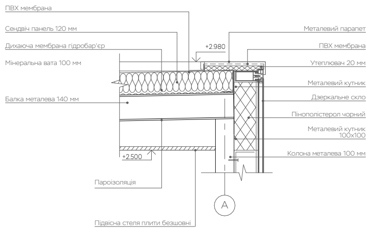
Вузол Б М 1:20
