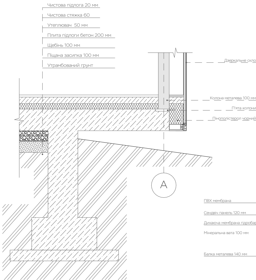
Вузол А М 1:20
