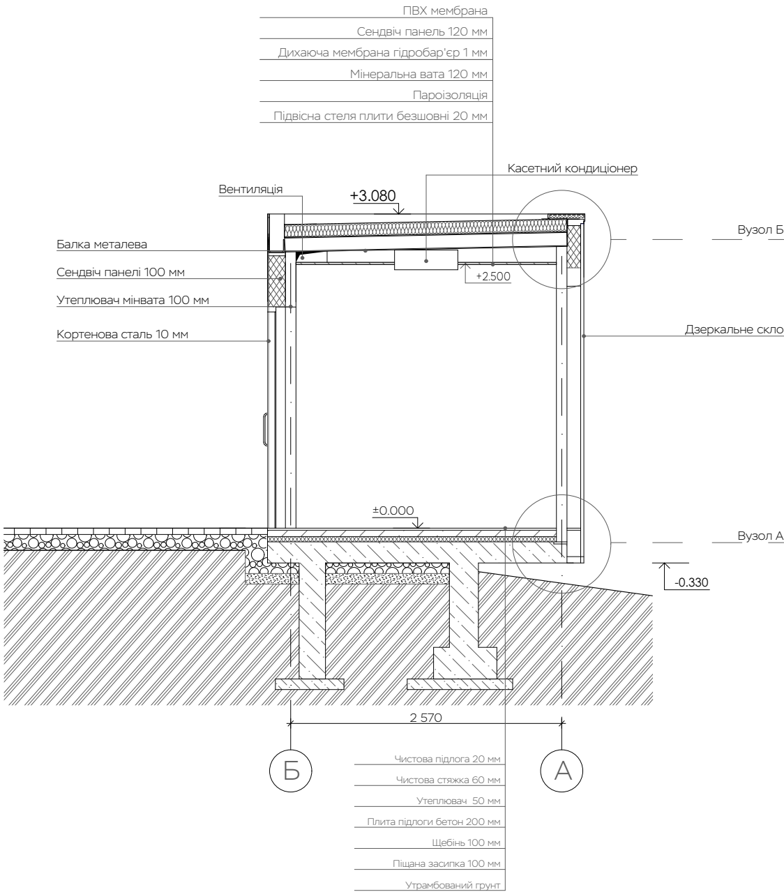
Переріз 2-2 М 1:50
