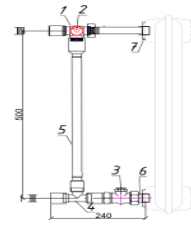
Байпас
